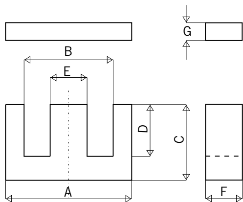
EI CORE
